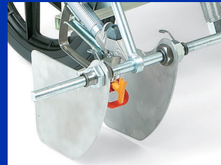
Protector de pulverización ajustable FieldLazer S100
